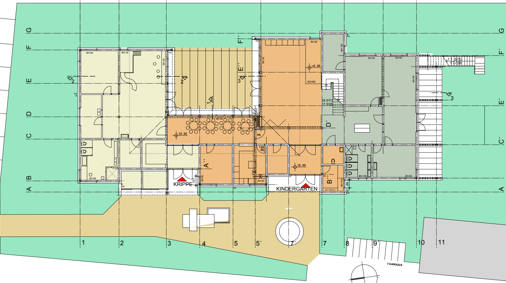
ERDGESCHOSS M. 1:200
